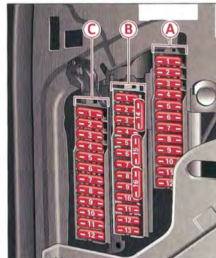
Fig. 184 Poste de conduite côté conducteur : porte-fusibles avec étrier en plastique (figure : véhicules avec direction à gauche)
