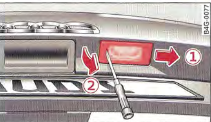
Fig. 212 Hayon : dépose du feu de plaque minéralogique
