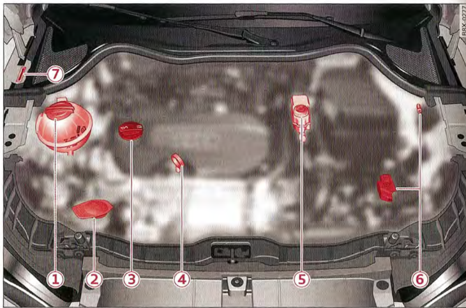
Fig. 148 Agencement des réservoirs, de la jauge d'huile-moteur et de l'ajutage de remplissage d'huile-moteur
