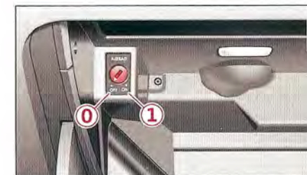
Fig. 127 Boîte à gants : commande à clé permettant de désactiver l'airbag du passager avant
