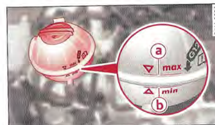
Fig. 152 Compartment-moteur : repères sur le vase d'expansion de liquide de refroidissement
