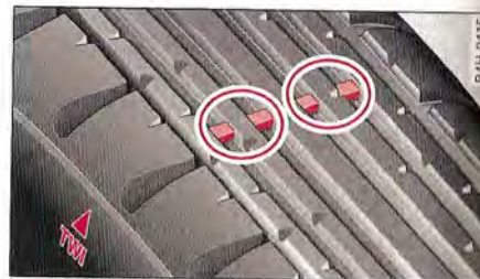
Fig. 159 Sculptures : indicateurs d'usure
