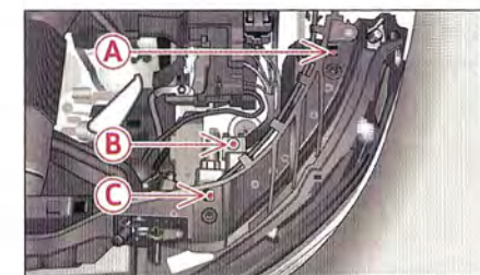
Fig. 201 Phare avant : points de fixation
